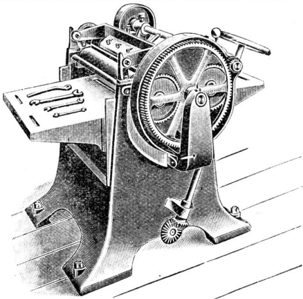
Dickehobelmaschine.
