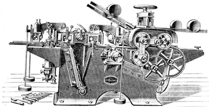
Schwere, vierseitige Hobelmaschine.
