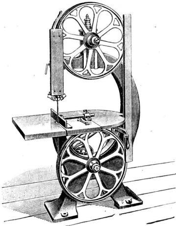
Kleinere Bandsäge.
