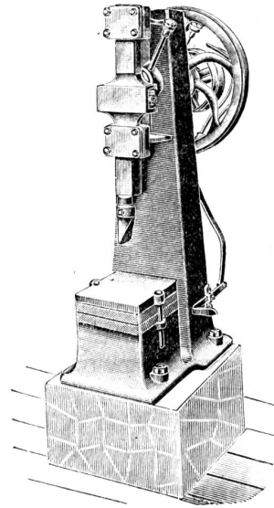
Holzspaltmaschine.
