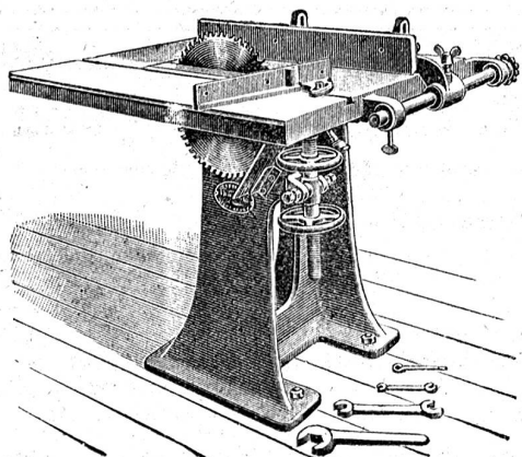
Kreissäge
