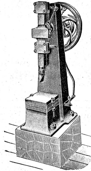
Holzspaltmaschine.
