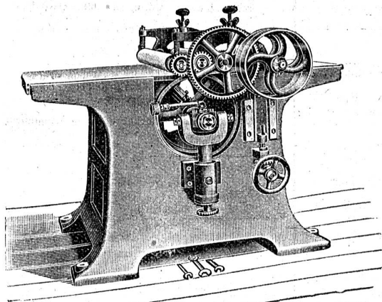
Sandpapierschleifmaschine.
