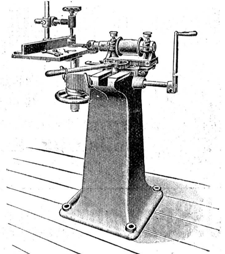
Langlochbohrmaschine.
