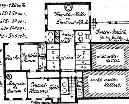
Keller.
