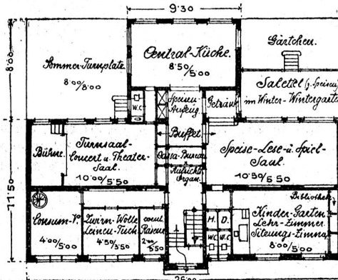
Parterre.
