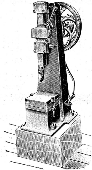
Holzspaltmaschine.
