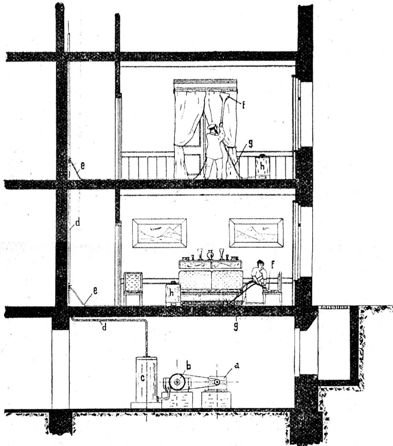
Durchschnitt eines modernen Hauses mit Vorfisg-Entstaubungsanlage (Maschinenanlage im Keller).
