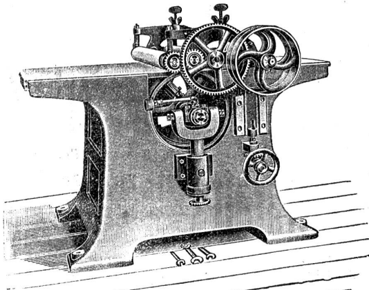
Sandpapierschleifmaschine.
