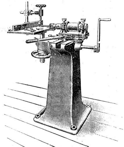
Langlochbohrmaschine.
