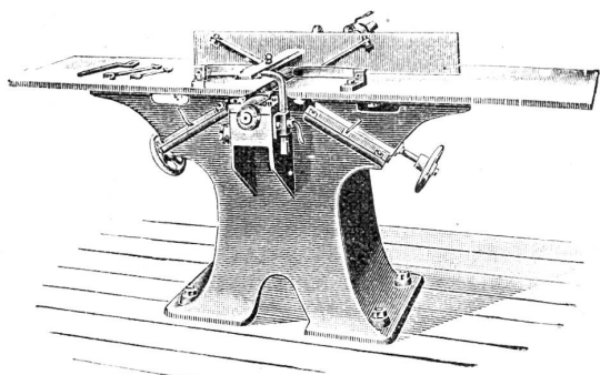
Abrichtmaschine.
