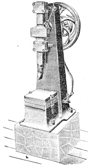
Holzspaltmaschine.
