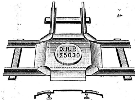
Fig. 2. Kletterwendepatte.
