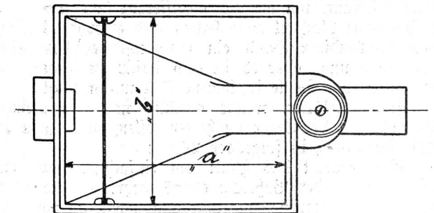
Fig. 3. Draufsicht.
