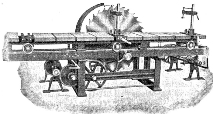
Kantholz- und Besäum-Kreissäge.
