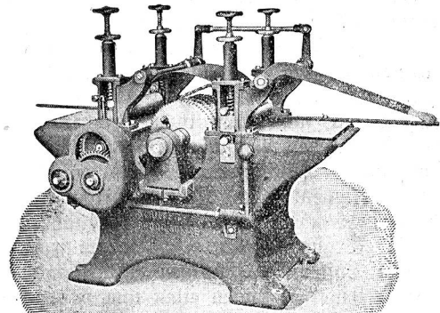
Latten-Kreissäge
