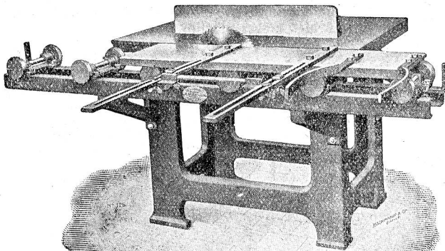
Kantholz- und Besäum-Kreissäge.
