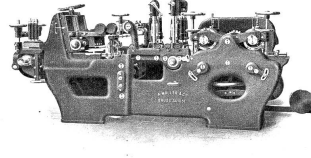
H. O. Große Hobel- und Kahlmaschine mit 4 oder 5 Messerwellen und horizontalen Palmenrollen, 500 und 600 mm Durchmesser.
