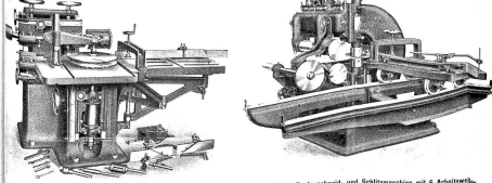
C. M. Kombinierte Zapfenstock- und Kahlmaschine mit Kahlwellen, 2 Messerwellen und Abkrügsäge, Pat. No. 49541. C. D. Zapfenstock- und Schlittenmaschine mit 4 Arbeitswellen.
