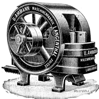
3330] Stationärer Brecher.
