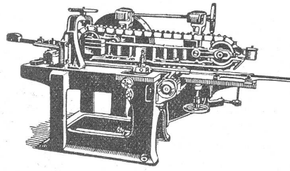
Vierseitige Parketthobelmaschine
