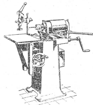
Riemenlose Langlochbohrmaschine
