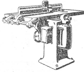
Riemenlose Präzisions-Kreissäge
