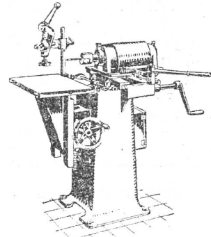
Riemenlose Langlochbohrmaschine
