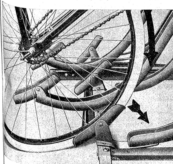
Fig. 3. Automatische Patent-Einfahrbrücken
