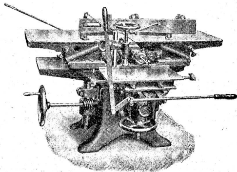
UNIVERSAL - KOMBINIERTE HOBELMASCHINE N. E. K. mit Kreissäge und Bohrmaschine 16 3
