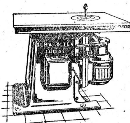
Riemenlose Kehlmaschine
