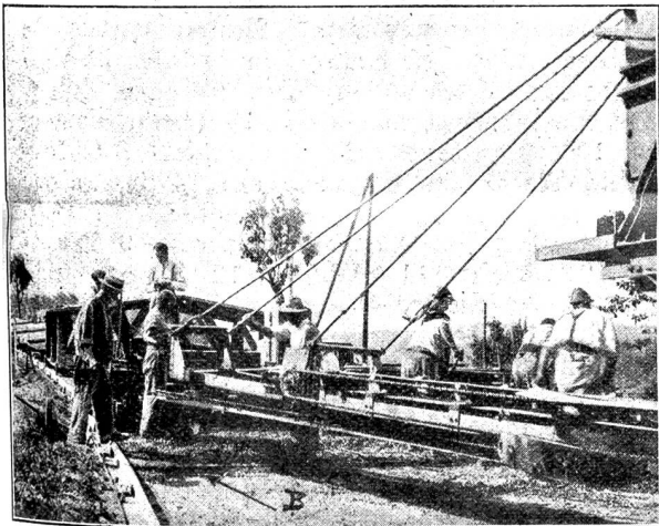
Abb. 6. Mischmaschine, Straßenfertiger in Tätigkeit, quer zwischen den Lauffschienen das hochgestellte Fugenbrett B.
