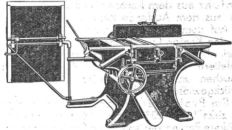
KOMBINIERTE HOBELMASCHINE — Mod. H. D. L. 410, 510, 60 mm Hobelbreite 23
