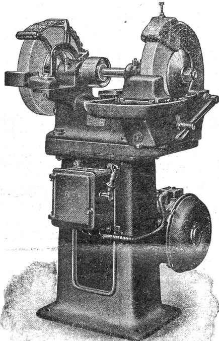
Mod. 30 b mit Einzelantrieb für Scheiben von 350×60 mm
