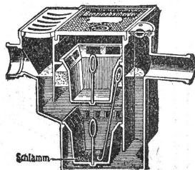
BENZIN-ABSCHIEDER
