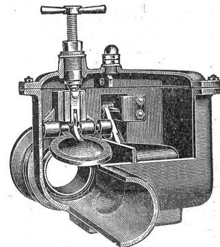
RÜCKSTAU-ABSCHLUSS
