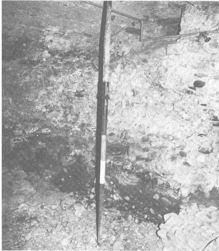
Abb. 37 Kaiseraugst, Dorfstrasse, Parz. 92. Turm 10, Nordwand des Kellers. Über dem gewachsenen Boden bilden schräg gesetzte Kieselbollen die Unterlage für das Turmfundament, in dem Spolien vermauert wurden. Darüber folgen mit Kieselbollen vermischte Kalkbruchsteinlagen. Ansicht von Südosten.
