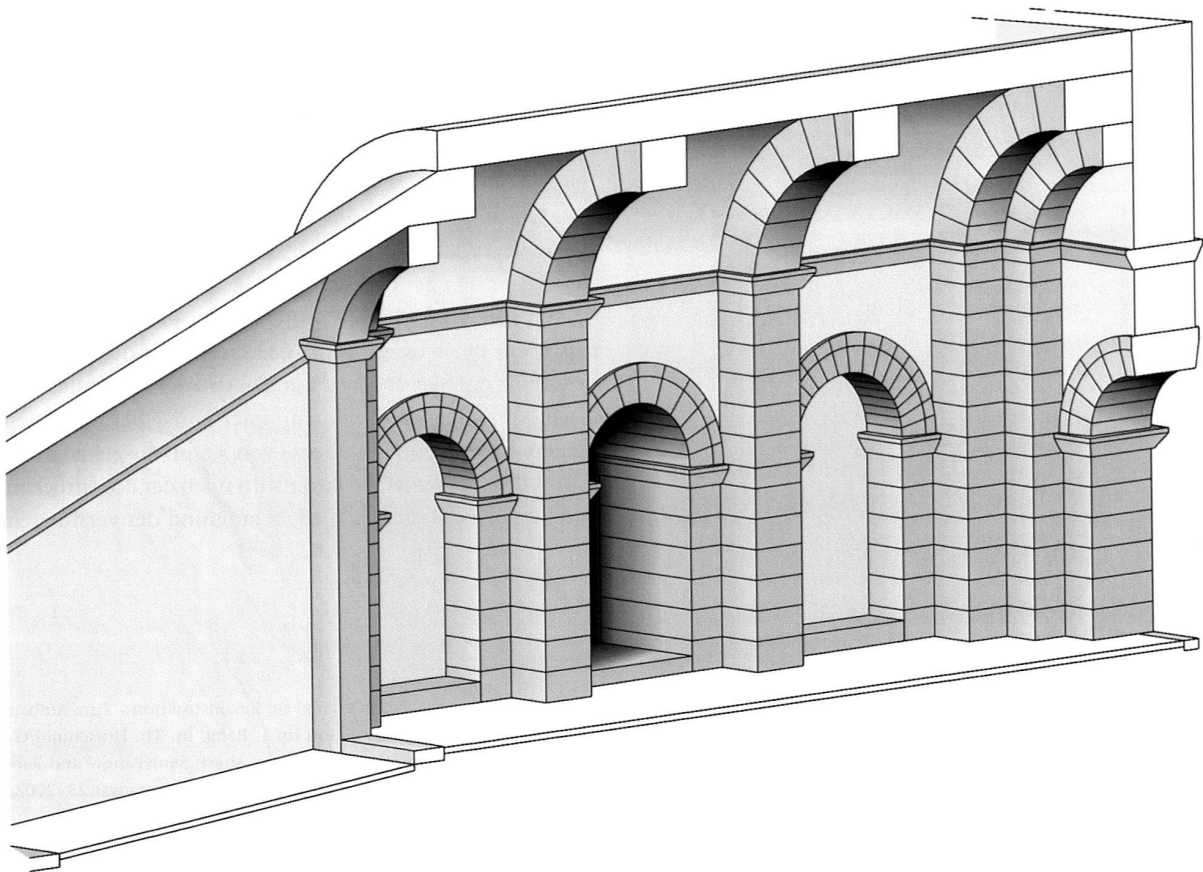
Abb. 10: Augst, Theatersanierung (Grabung 2002.S5). Blendbogen der südlichen Eingangshalle. Rekonstruktionsversuch der östlichen Hallenwand mit Durchgangsbogen zum so genannten südlichen Treppenhaus in der Mitte und zwei seitlichen Blendbogennischen. (Das 2002 gefundene, abgestürzte Mauerstück [Abb. 2–9] gehört zur südlichen Nische, rechts im Bild.) Gut erkennbar ist auch das Grundgerüst der Hallenkonstruktion, bestehend aus vorkragenden Gurt Pfeilern und Gurtbögen (aus massiven Buntsandsteinblöcken) und einem darüber liegenden Tonnengewölbe (vermutlich aus Kalktuffquadern). Der von Süden her (ganz rechts im Bild) in die Halle führende Durchgang ist hypothetisch, ergibt sich aber aus der Logik des Grundrisses und in Übereinstimmung mit vergleichbaren Bauten. Isometrische Ansicht unmassstäblich.
