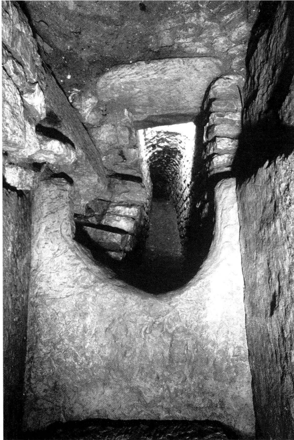
Abb. 24: Augst, Theatersanierung (Grabung 2002.55). Abwasserkanal, Verzweigung im Süden, südöstlicher Abschnitt mit Sandsteinkammer. Blick von Nordwesten, von der Sandsteinkammer aus in den südöstlichen Fortsetzungskanal. Im Zentrum die U-förmig ausgehauene Mündung; in der oberen Bildhälfte der Sandsteinarchitrav mit dem Entlastungsbogen aus Buntsandsteinecken (vgl. Abb. 27). Links der verstürzte Sandsteinarchitrav des von den Frauenthermen her kommenden, nordöstlichen Seitenkanals (vgl. Abb. 29).
