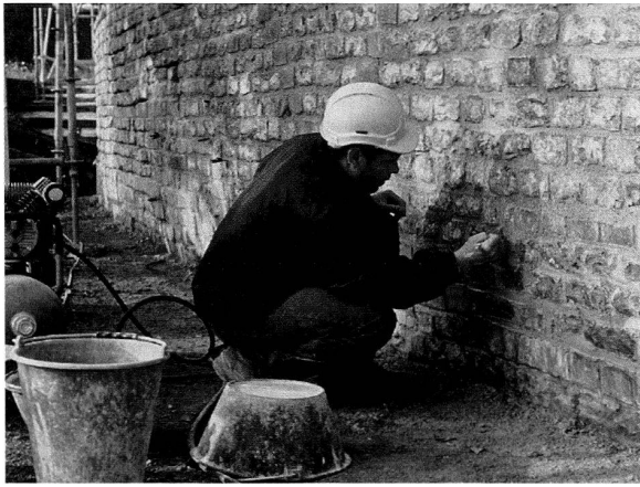
Abb. 41: Augst, Theatersanierung (Grabung 2002.55). Sanierungsarbeiten an der Peripherie von Keil 2. Arbeiter Salim Leghdesmi beim Neuverfugen der Mauerschalen.
