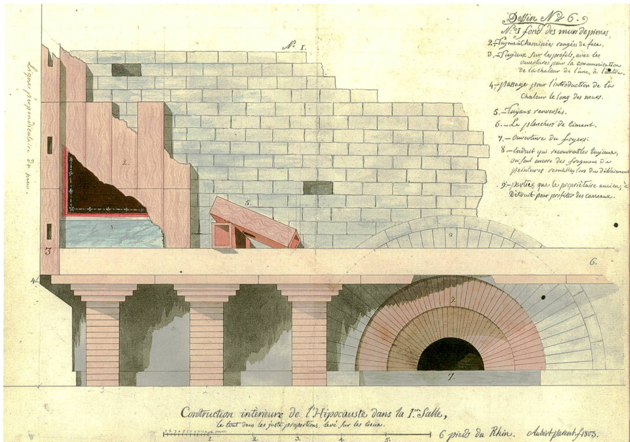
Abb. 17: Augst BL, Heilbad in der Grienmatt (Grabung 1803.062). Idealisierte Darstellung der im Tepidarium vorgefundenen Hypokaustheizung.
