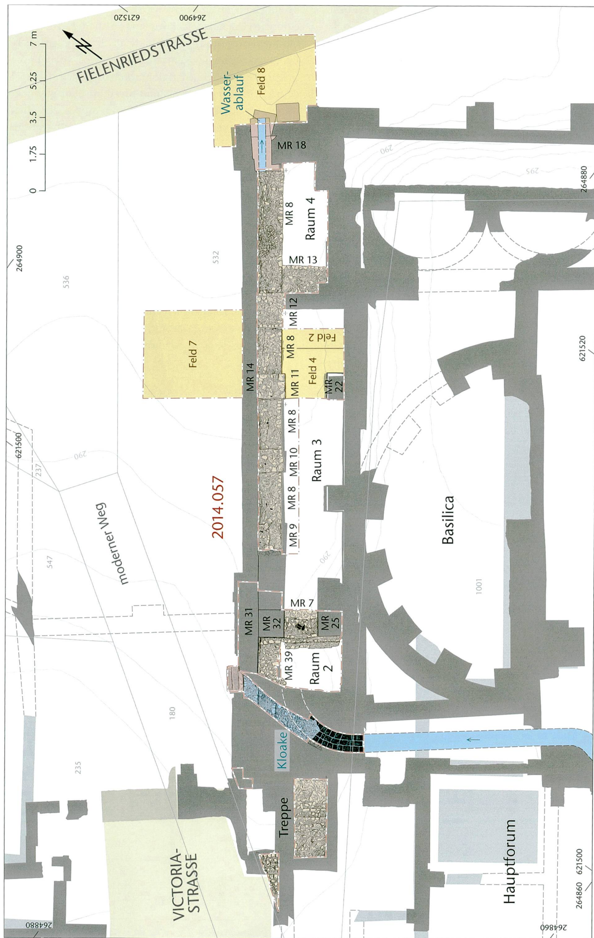
Abb. 49: August BL, Stützmauern Basilica (Grabung 2014.057). Situationsplan mit jenen Mauer-, Feld- und Raumnummern, die im Text erwähnt werden. Die anderen Mauerzüge sind summarisch dargestellt. M. 1:175.
