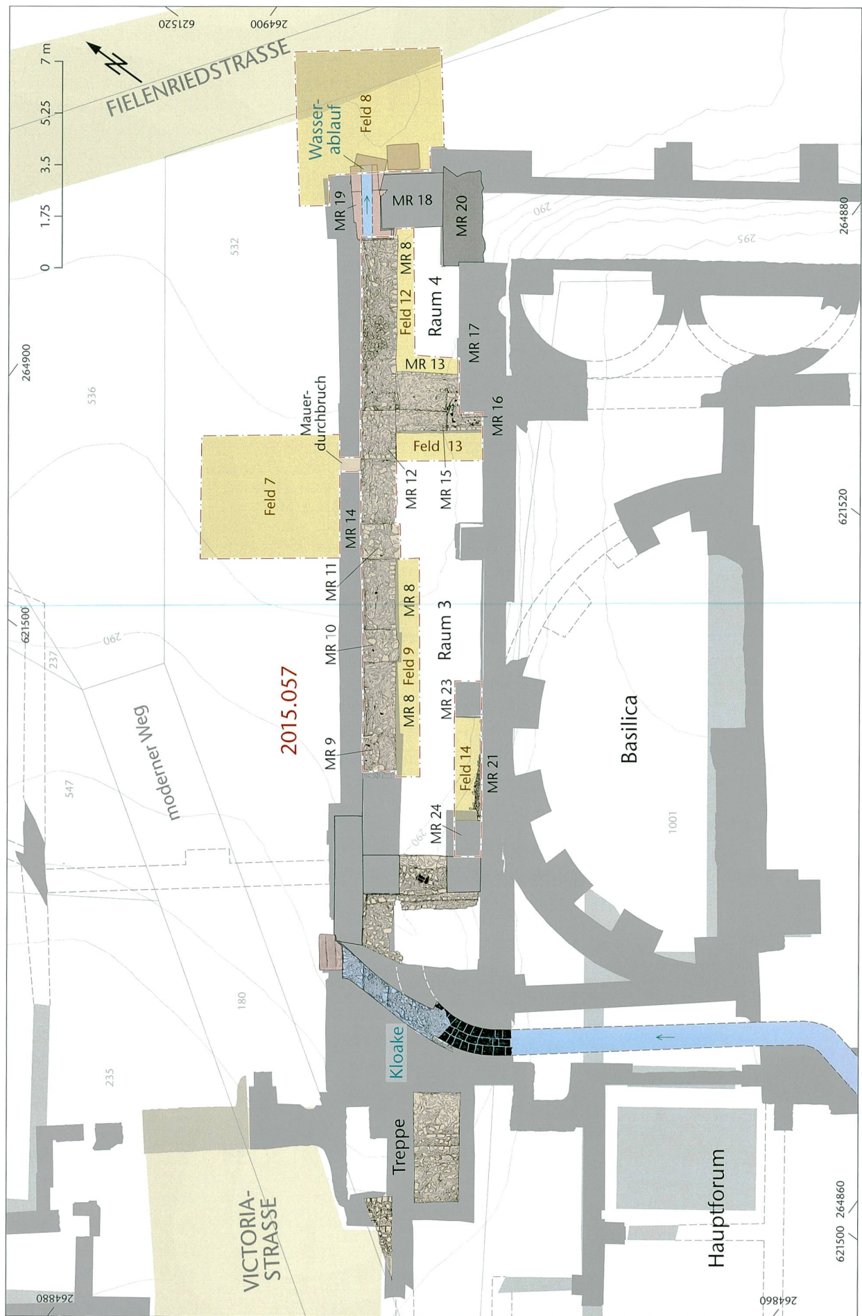
Abb. 50: August BL, Basilica-Stützmauern (Grabung 2015.057). Grundrissplan des sogenannten Treppenhauses. Eingetragen und angeschrieben sind die im Berichtsjahr tangierten Mauern und die Grabungsfelder, in denen Abtragsarbeiten durchgeführt wurden. M. 1:175.
