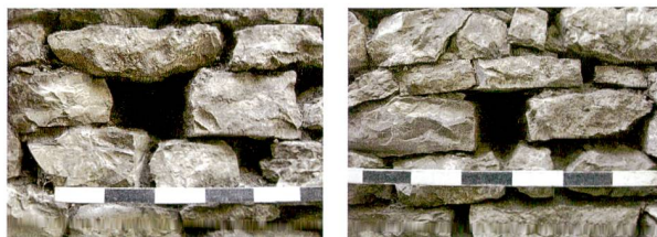
Abb. 8: Kaiseraugst AG, Auf der Wacht (Grabung 2011–2013.001). Schacht MR 6/MR 32 (Zustand im März 2016). Mit modernen Holzbalken markierte Balkennegative in MR 32 und Detailaufnahmen der beiden Balkennegative (vgl. dazu auch Abb. 9).
