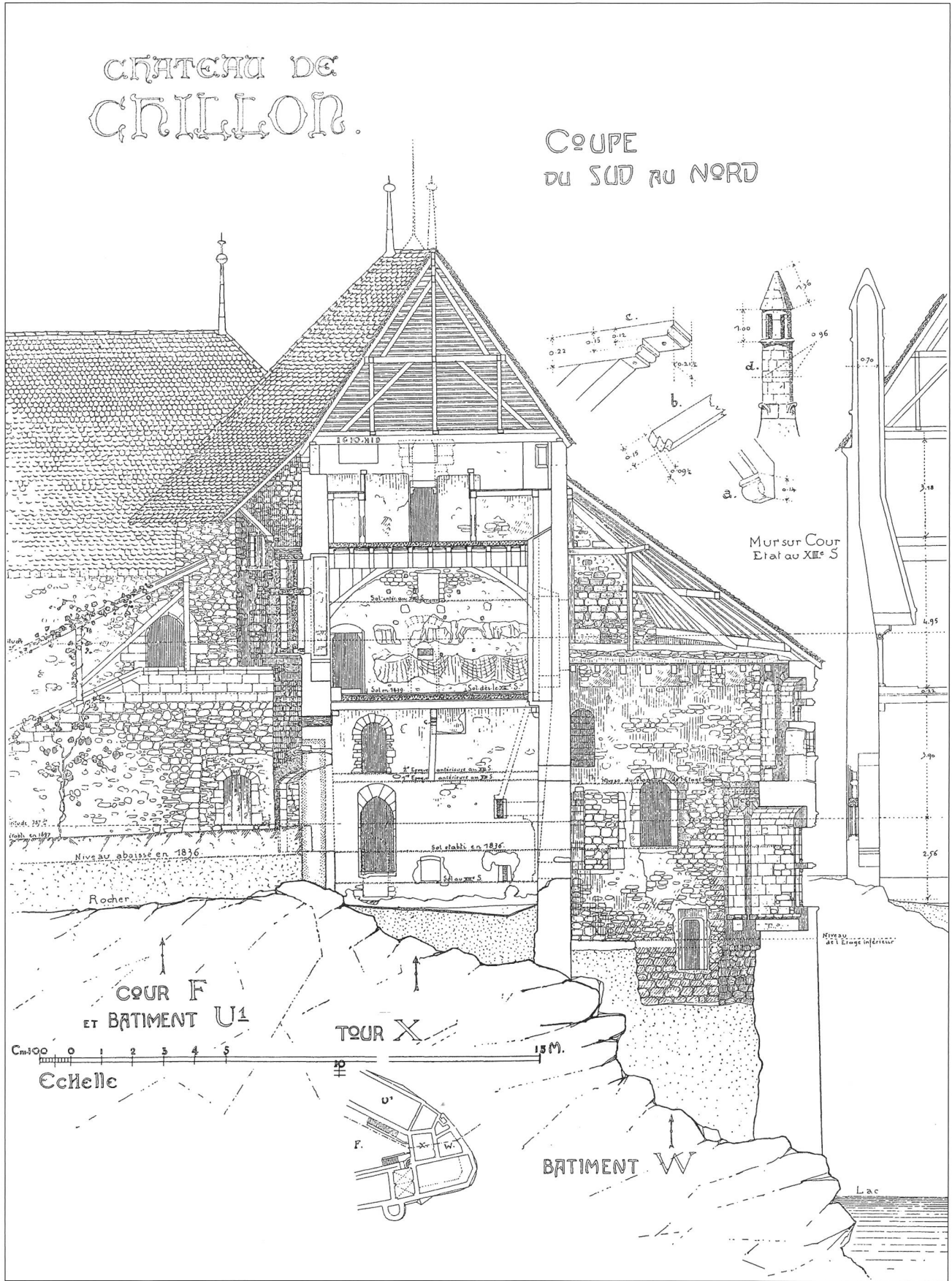
Fig. 13. Veytaux VD, Château de Chillon. Coupe du Sud au Nord. De : Naef 1908, pl. 4.
