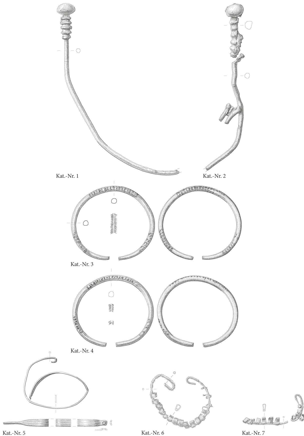
Abb. 15. Wagenhausen TG Etzwilen, Tättbüel. Nadeln, Armringe, Blecharmband, Drahtgehänge. M. 1:2. Zeichnung AATG, J. Näf.
