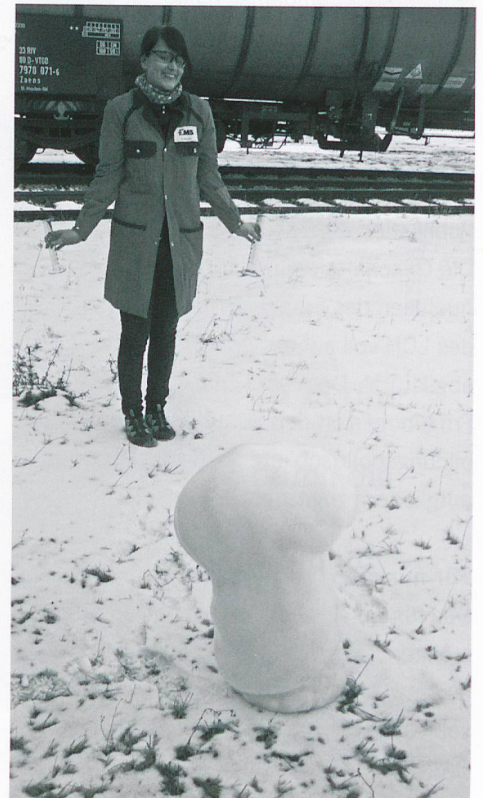
Aus Wasserstoffperoxid, Kaliumiodidlösung sowie Spülmittel lässt sich eindrucksvoll «Elefantenzahnpasta» herstellen.
