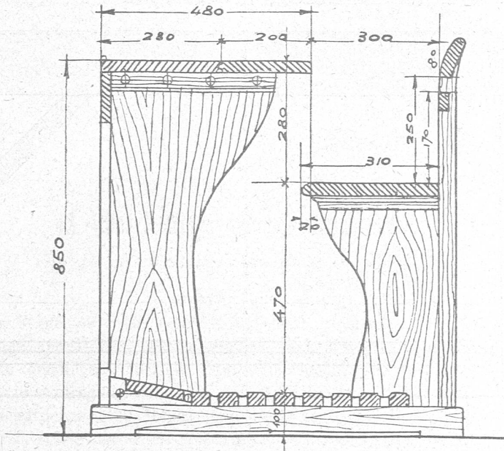
Querschnitt.
