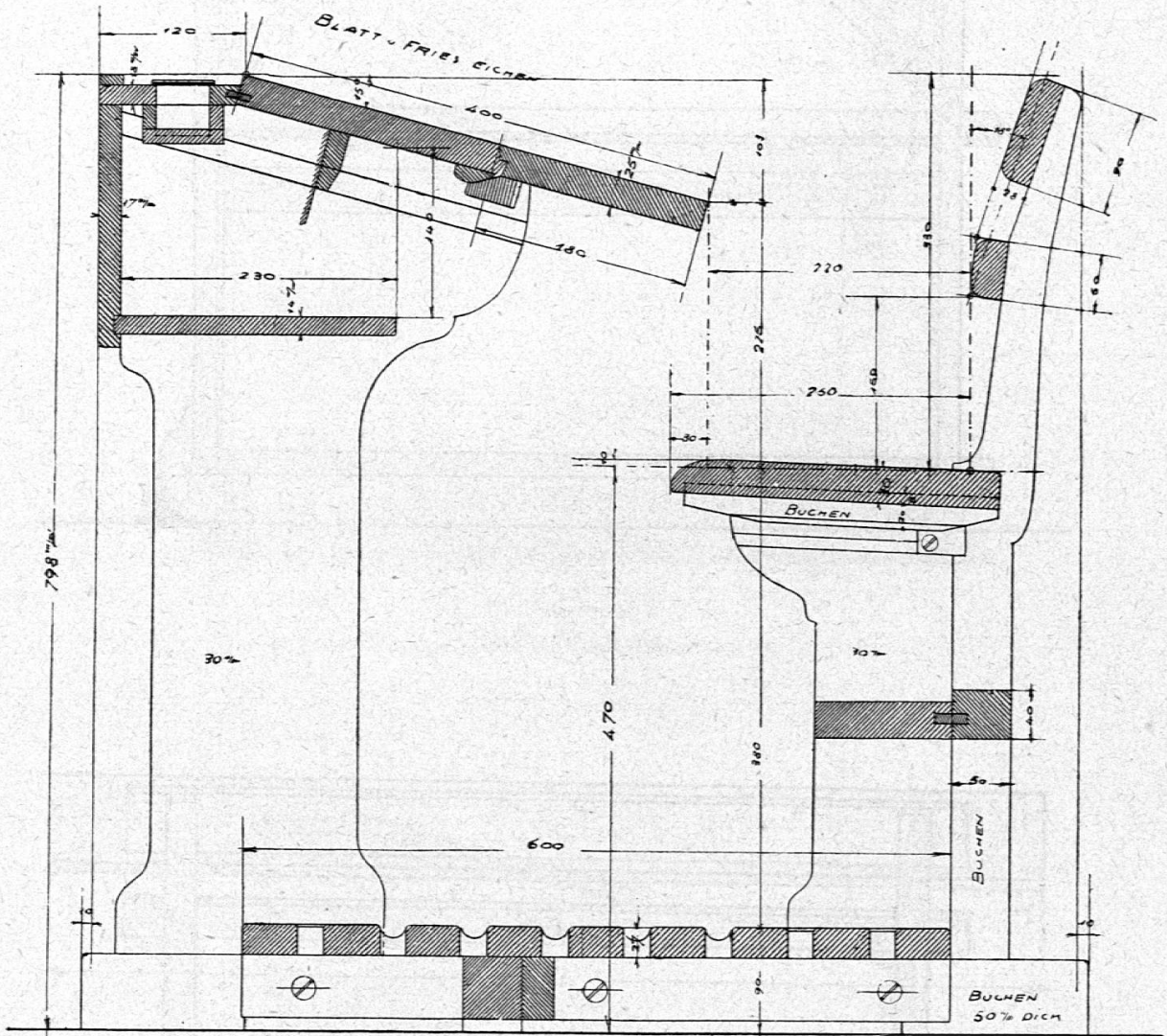
Seitenansicht mit Massangabe. No. 4.
