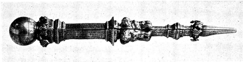
Abb. 5. Astronomisches Universal-Instrument aus Silber, dat. 1578.
