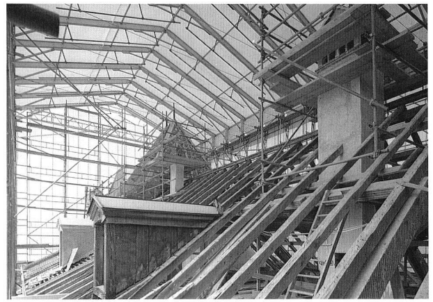
Fig. 11. La charpente découverte protégée par le toit provisoire. Photo Henri Germond, Lausanne.
