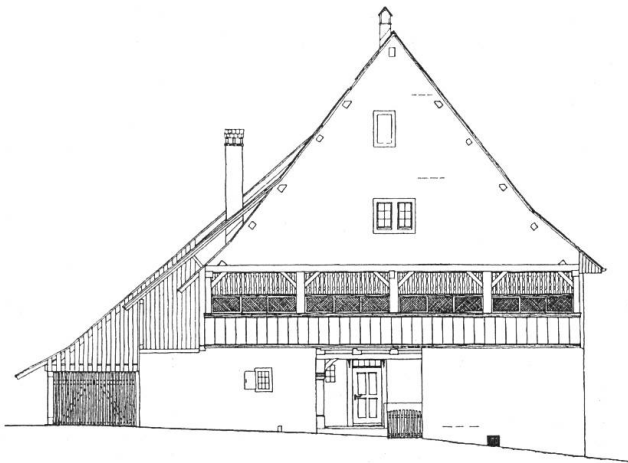
Giebelfassade
