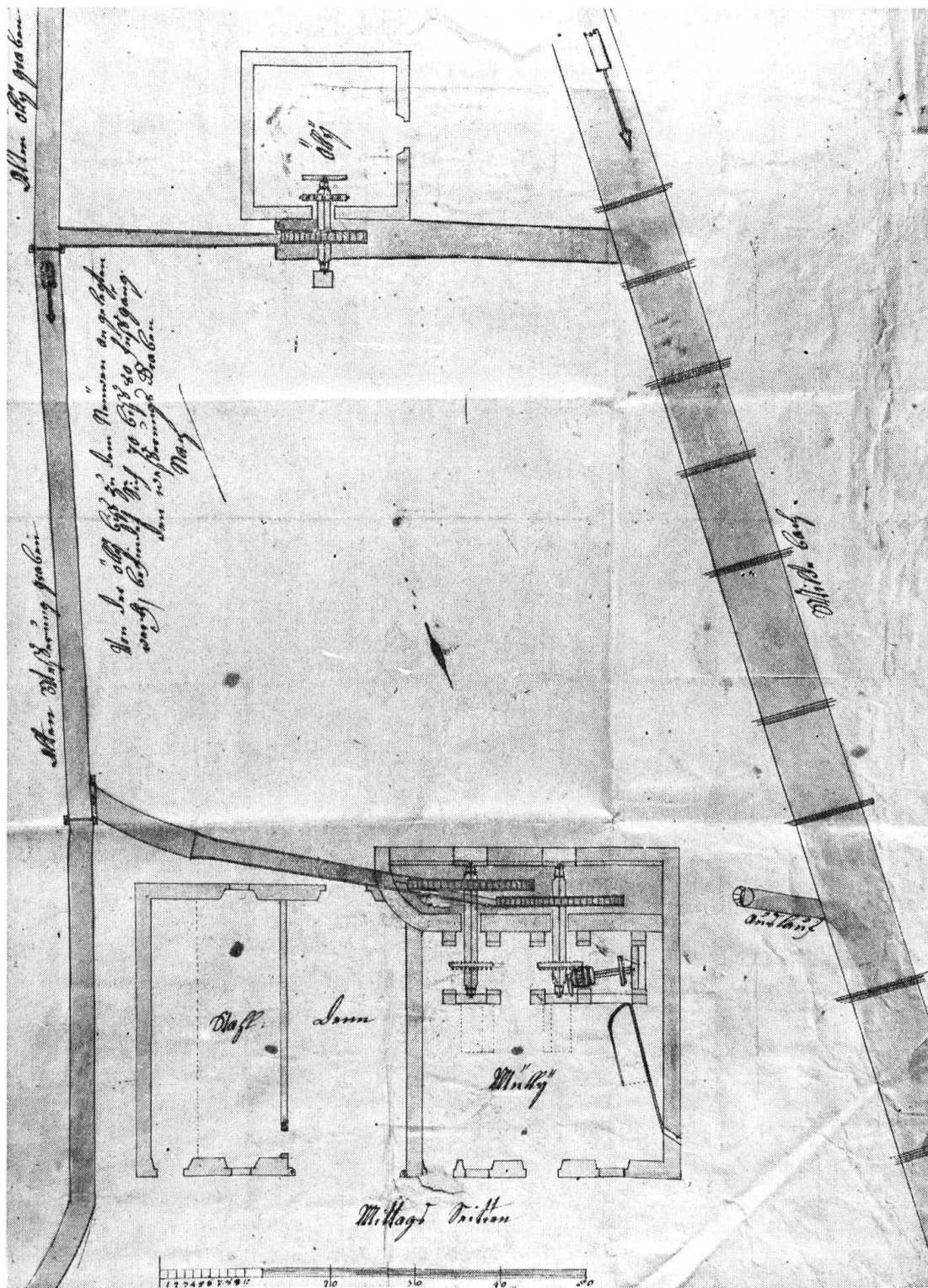
Plan der Adam-Mühle von 1800. Unten die projektierte Mühle, oben die bestehende Öl.
