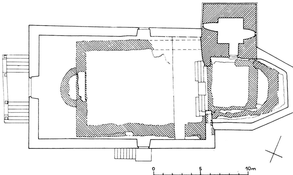
Archäologischer Grundriß von St. Pankraz
