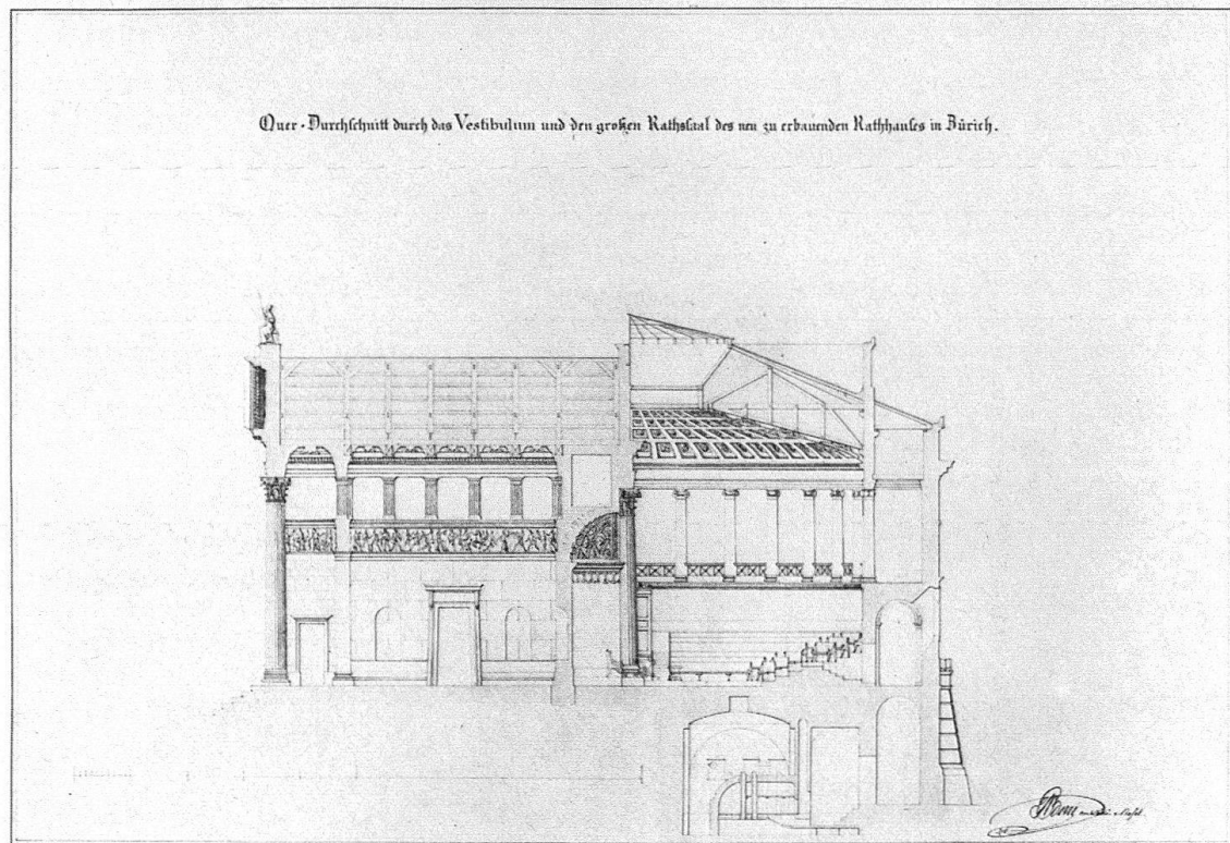
Abb. 7, 8. Melchior Berri (1801–1854): Baurisse für ein Grossratsgebäude, 1832 (Basel, Kupferstichkabinett)
