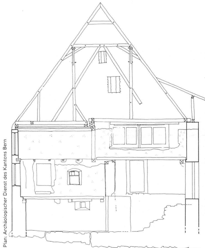
Unterseen, obere Gasse 42, Querschnitt durch das spätgotische Haus
