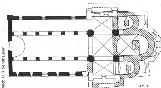
Rougemont, Kirchengrundriss
