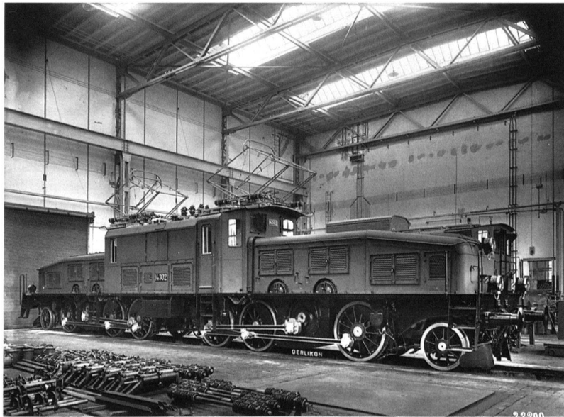
Lokomotive ICC1, Nr. 14302 der SBB im Verkehrshaus der Schweiz in Luzern.
