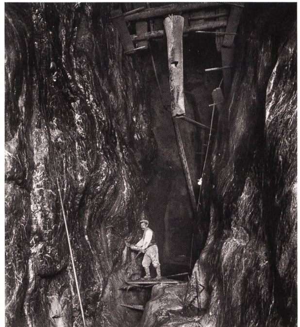
Für eine solide Fundierung der Staumauer im festen Fels waren im Schräh umfangreiche Aushubarbeiten notwendig.
