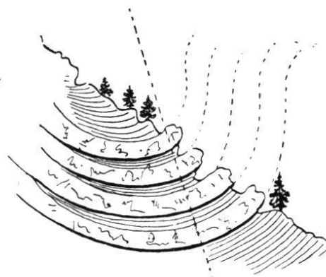
Schiefe Muldenare
