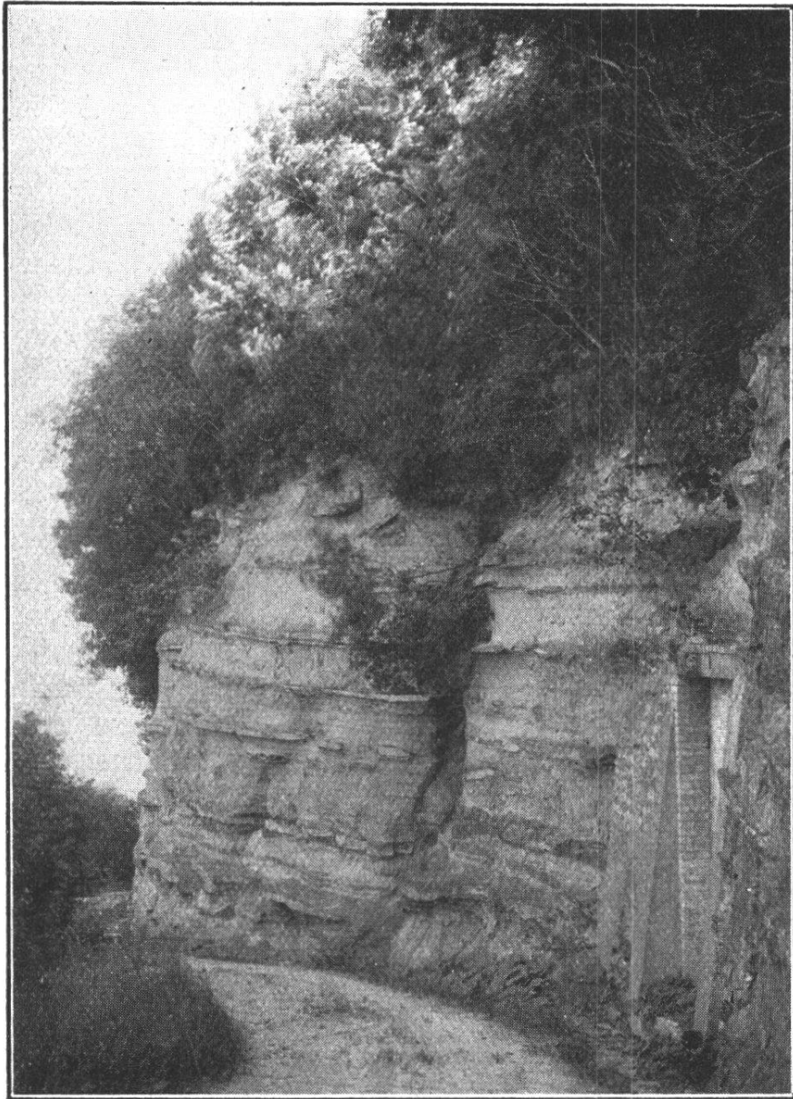
Fig. 9. Molasse marine (Burdig.)
