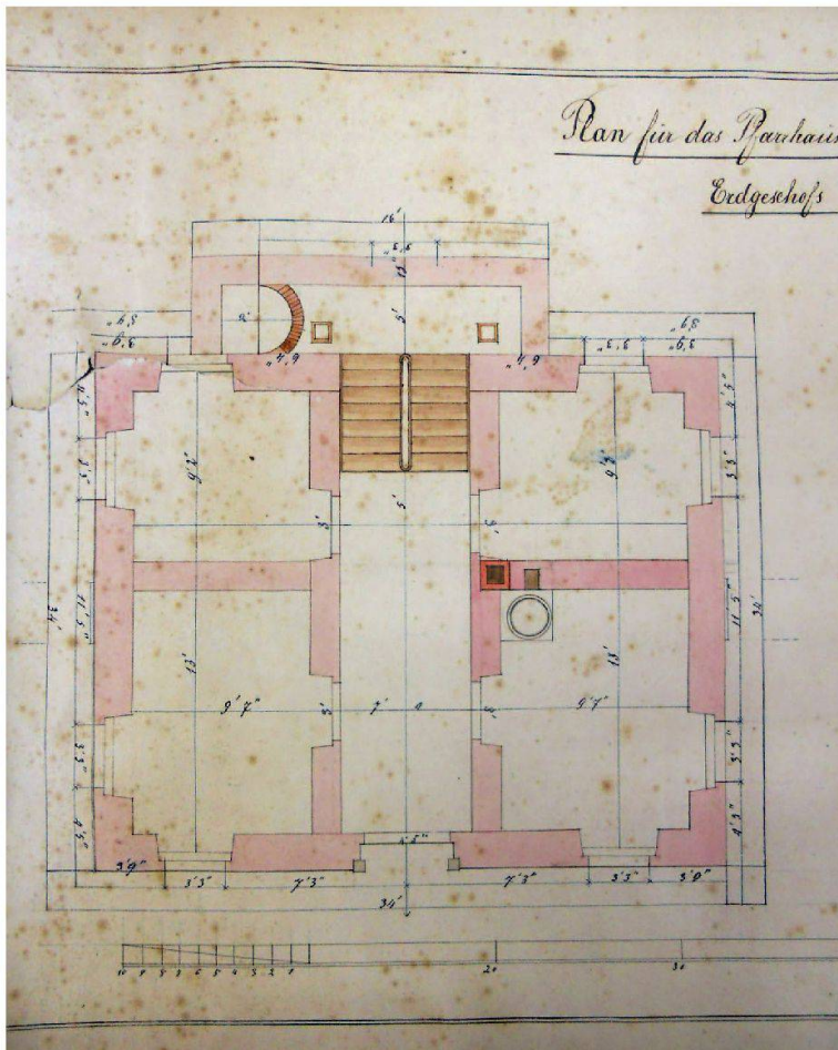
Abb. 4: Im Pfarrarchiv Alpthal hat sich nicht nur zur Pfarrkirche, sondern auch zum Pfarrhaus ein erstaunliches Konvolut an Bauplänen erhalten. Diesen Ausführungsplan signierte der Einsiedler Förster, Zimmer- und Baumeister Zacharias Kälin am 6. April 1878. Der 1880 vollendete Bau ist wie die drei Gasthäuser Sternen, Mythen und Schäfli im Stil eines Zimmermeisterhauses errichtet. Charakteristisch ist das hohe gemauerte Erdgeschoss mit Eingang an der traufständigen Hauptfassade. Darüber erhebt sich ein zweigeschossiger Blockbau mit Ecklisenen und eingemitteten Lukarnen. Rückseitig befindet sich das vorspringende Treppenhaus. Feder in Tusche und Aquarell über Bleistift auf Papier.
