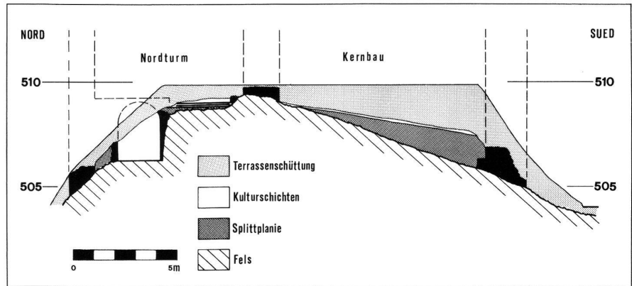
Querschnitt durch die Vordere Burg
