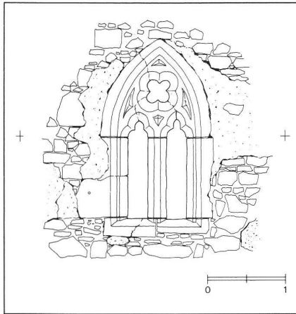
Neu-Thierstein 85 Fassade West, 3. Geschoss, Fenster Süd
