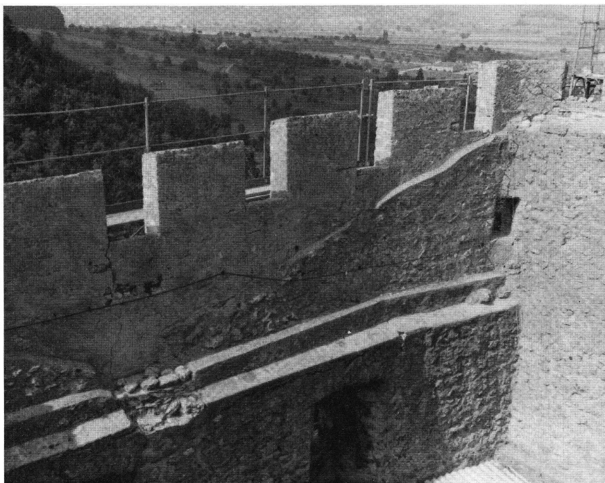
Neu-Thierstein, Inneres des Wobenturms. W-Mauer des obersten, nachträglich aufgesetzten Geschosses mit rekonstruiertem Zinnenkranz und V-förmigem Mauerabsatz für die doppelte, nach innen geneigte Dachschräge. Zustand 1984.
