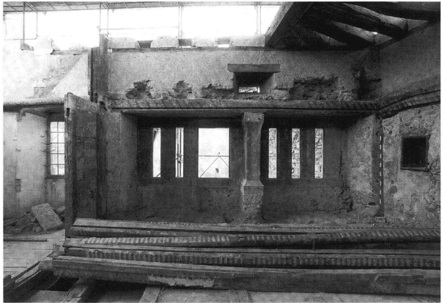
Palas von 1318. Truchsessensstube. Südwand mit Fensterscharten. Links Reste der Bohlenständerwand, die diesen Raum vom oberen Saal im Osten abtrennte. Über dem Sturz der Fensternische: Südwand des ehemaligen Blindbodens zwischen der Bohlen-Balken-Decke und der tragenden Balkenlage. Von dieser ist rechts oben noch der westliche Balkenfächer sichtbar, der den Palas-Obergaden im Westen trug. Links davon sind noch die Negative der beim Umbau von 1991 entfernten Balken zu erkennen.
